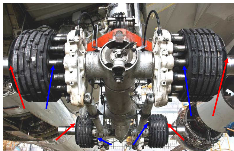
Sur la photo ci dessus les roues son démontées
