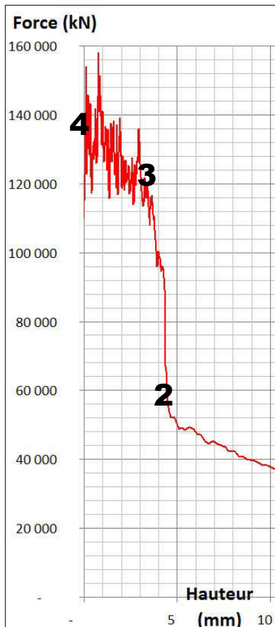
< Zoom de la courbe d'effort sur les 10 derniers mm de forgeage
